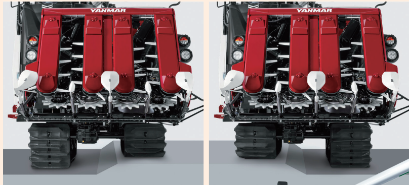
写真2 車体水平制御
