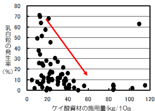
ケイ酸の補給によって乳白粒の発生率が低下する
