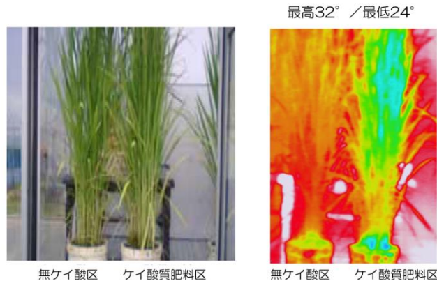
ケイ酸施用と高温化におけるイネの体温
