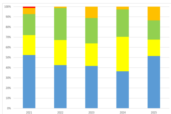
愛媛県 温州みかん pH の分布割合
