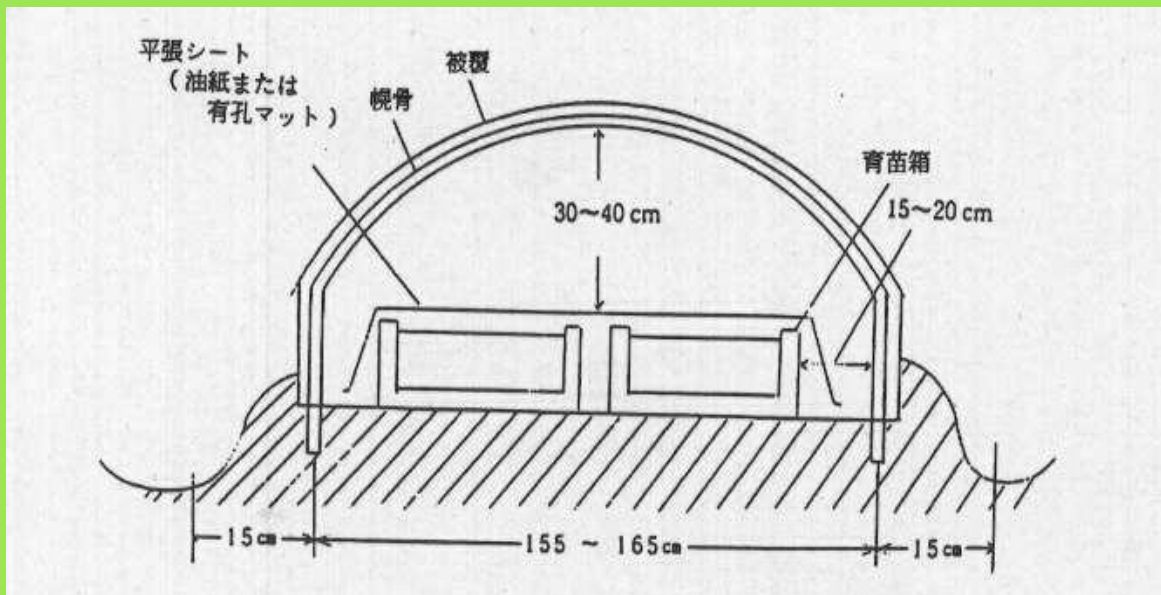
図 シルバーポリシートによるトンネル被覆の育苗図
