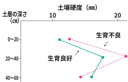
図-2 生育不良野菜畑の層別土壌硬度 注）土壌硬度は山中式硬度計で測定した
