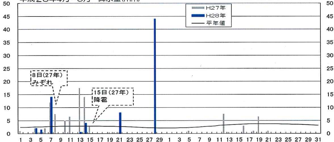
平成28年4月～5月 降水量(mm)
