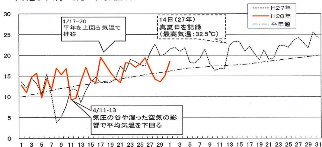
平成28年4月～5月 平均気温(℃)
