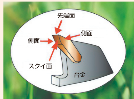
図2 「JAチップソー」のチップの特徴
