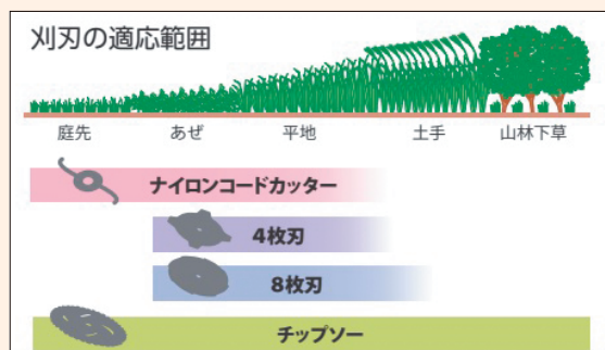
図1 刈払機に使用する刈刃の適用範囲
