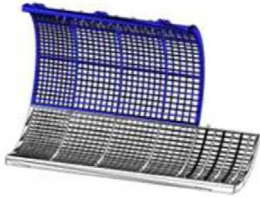
ステンレス製受網 (耐摩耗性の向上)
